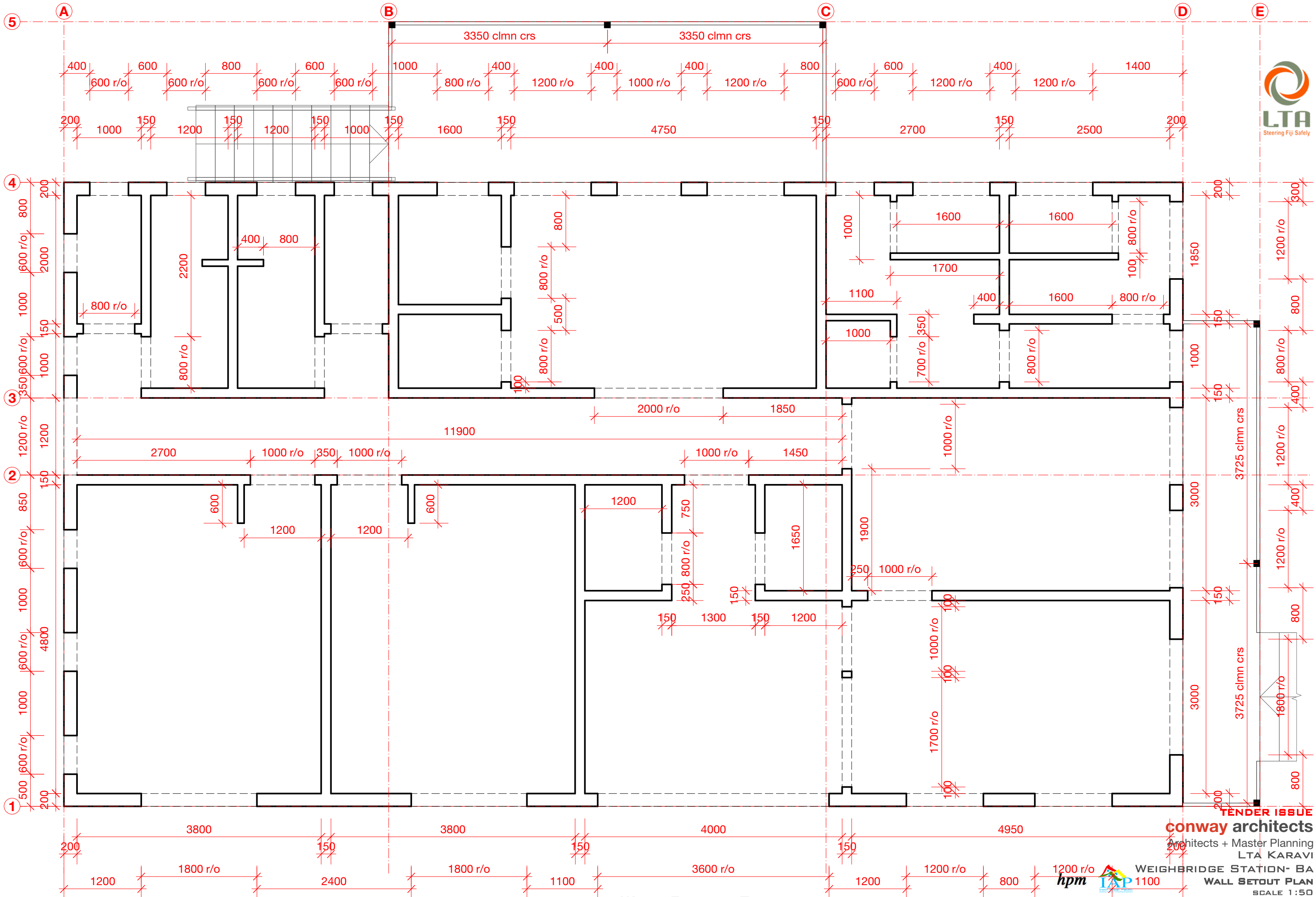
WALL SETOUT PLAN
