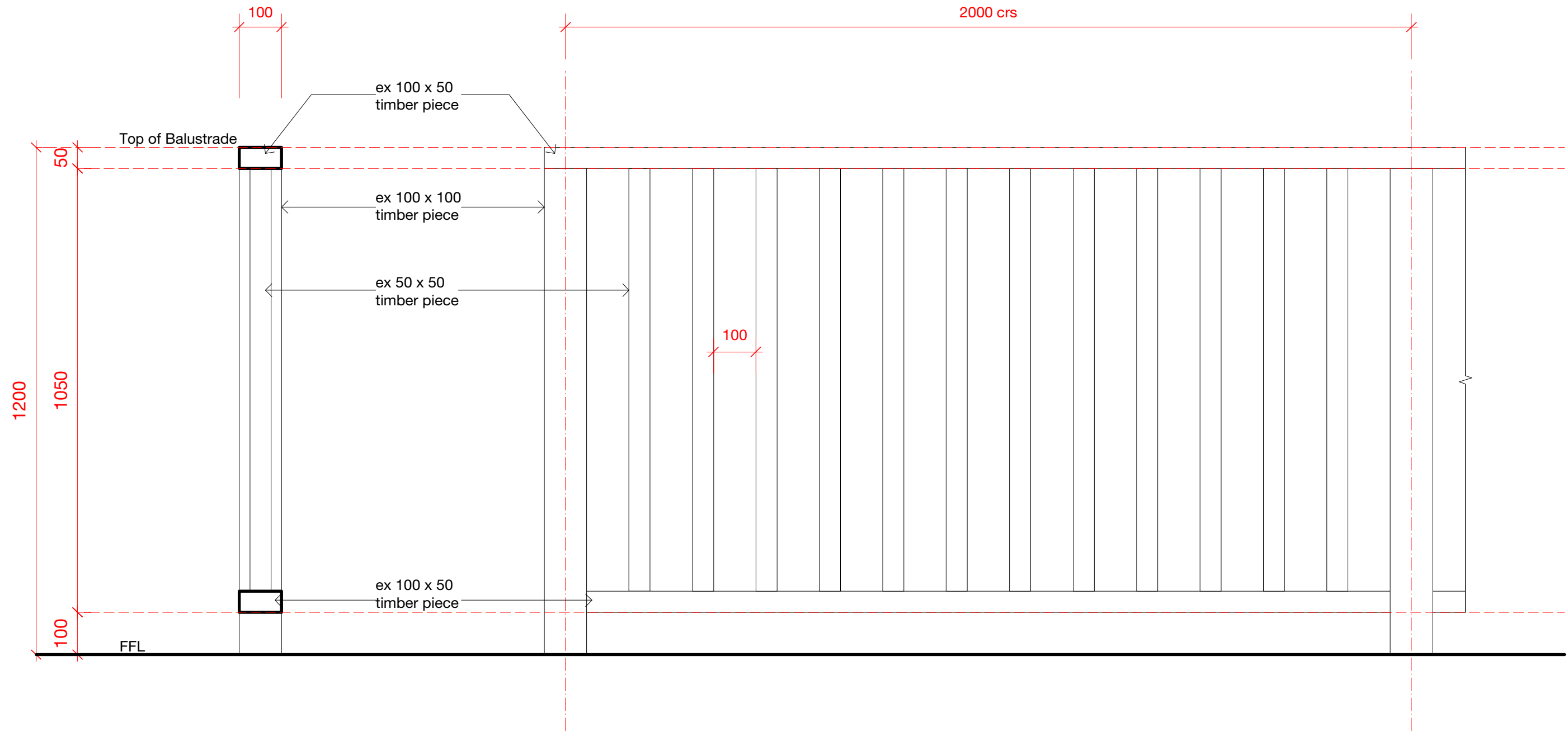
1 BALUSTRADE DETAIL 1 SCALE: 1:10
